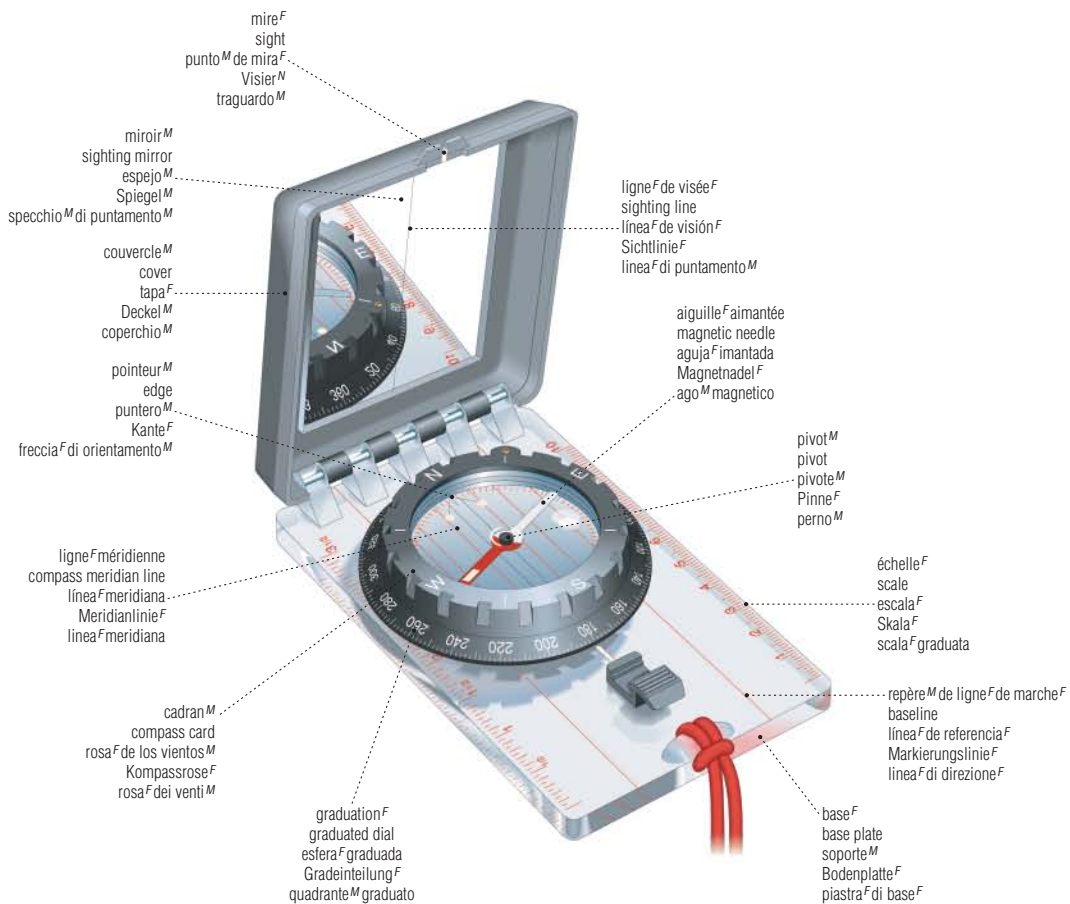
boussole F magnétique magnetic compass brújula F magnética Magnetkompass M bussola F magnetica
